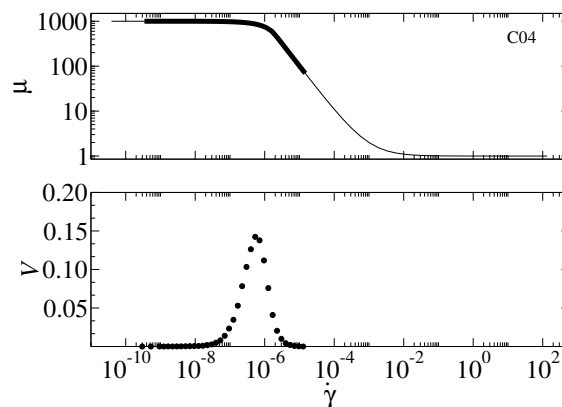
Figura 1: Comportamento da viscosidade e velocidade com a taxa de deformação do fluido.
