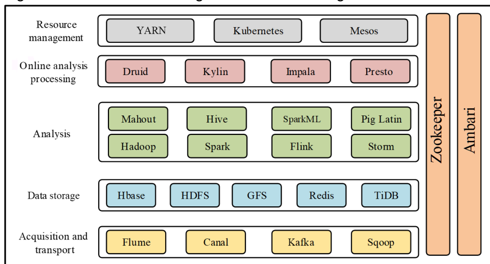
Figura 1 – Pilha de Tecnologias utilizadas em Big Data
